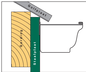
Aluminium dakgoot bevestigd aan de geprofileerde staalplaat.
