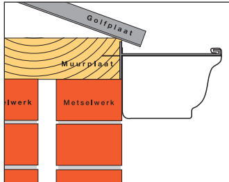
Gemonteerd aan de muurplaat met metselwerk.
