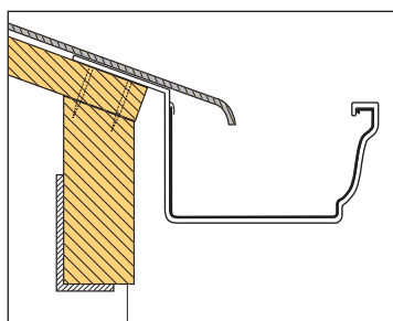
Aluminium dakgoot bevestigd aan het dakbeschot.
